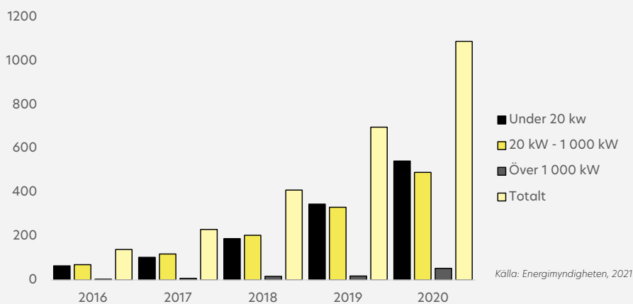
Figur 1 - Installerad effekt (MW)
